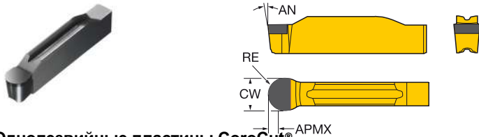
Однолезвийные пластины CoroCut®
